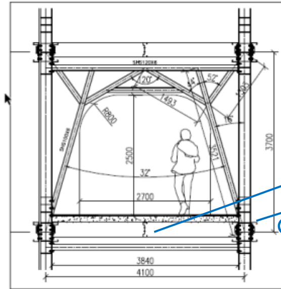
ALZADO G-G
